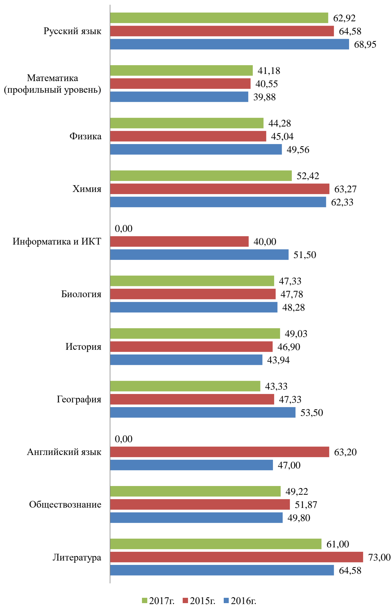
Диаграмма изменения среднего тестового балла по району (11 класс)
