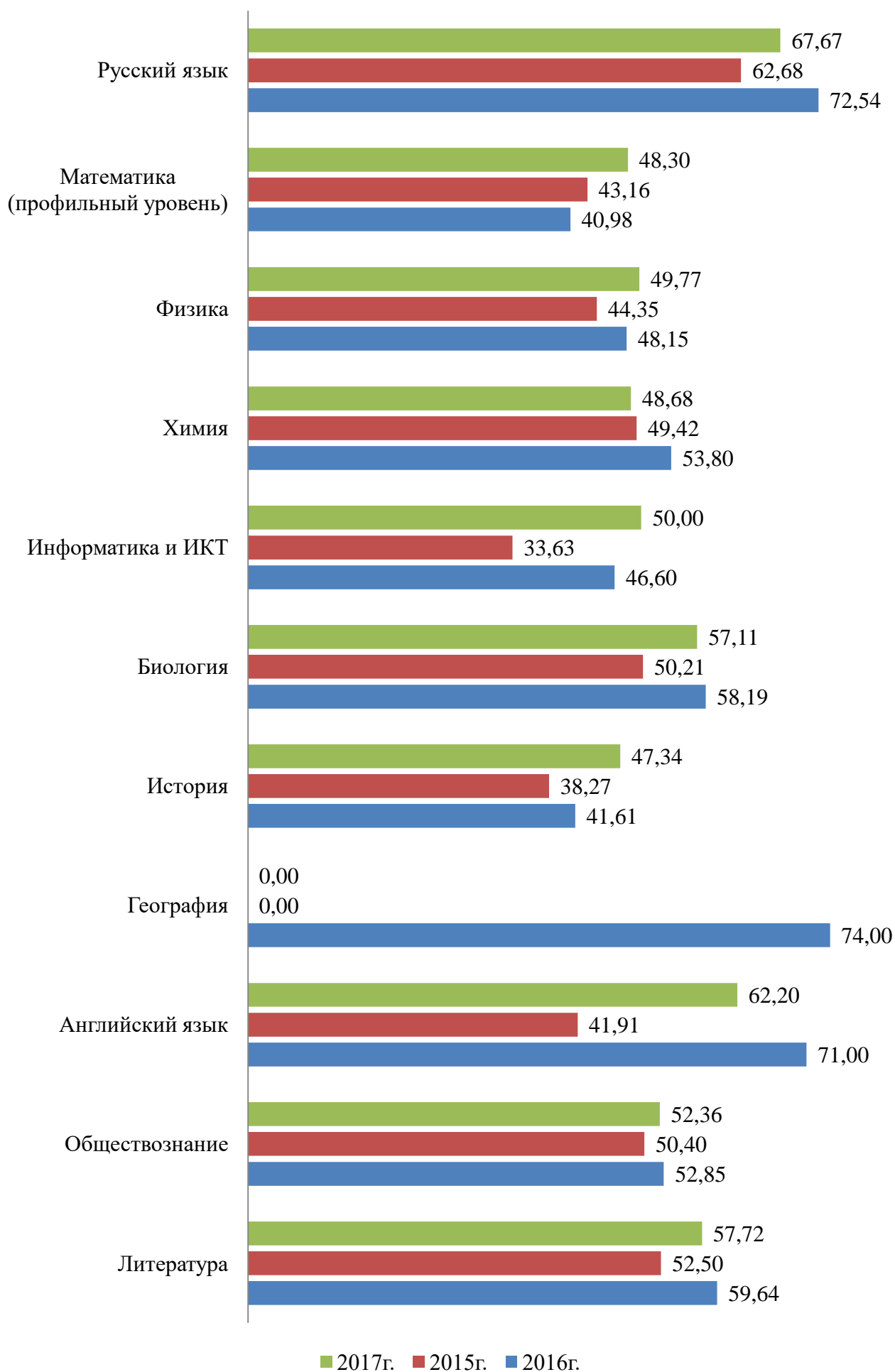
Диаграмма изменения среднего тестового балла по городу (11 класс)
